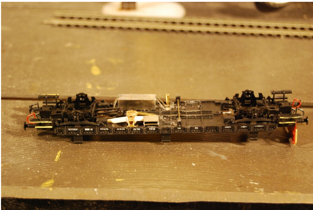
Bildet viser korrekt plassering av av Schweitzerapparat og batteriboks for vognene 19900-19912. Bremsedelene er ikke montert på dette stadiet.
