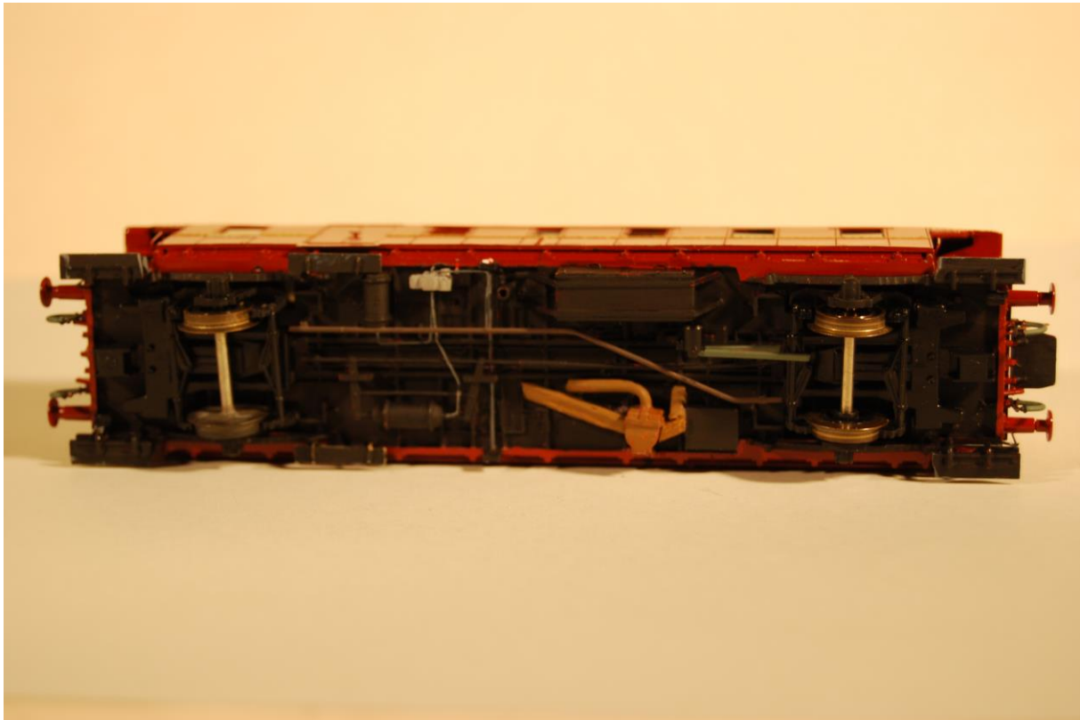
Bildet viser korrekt plassering av alle understellsdeler ifor vognene 19913-19921
