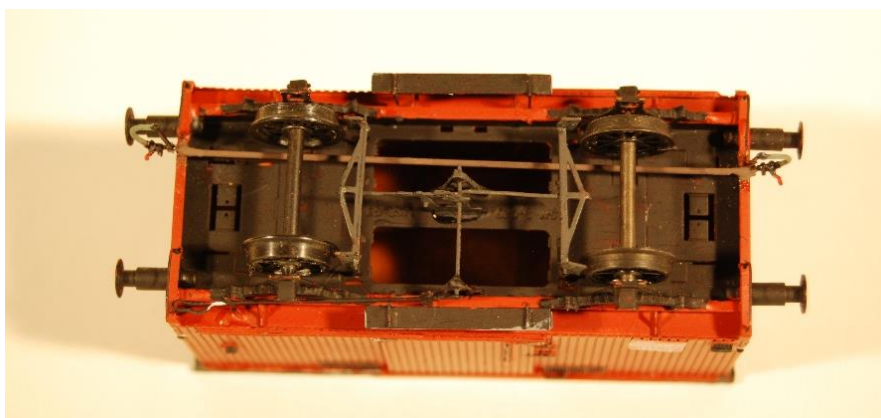
Bildet viser en G3 vogn men prinsippet for montering av gjennomgående bremsledning er det samme
