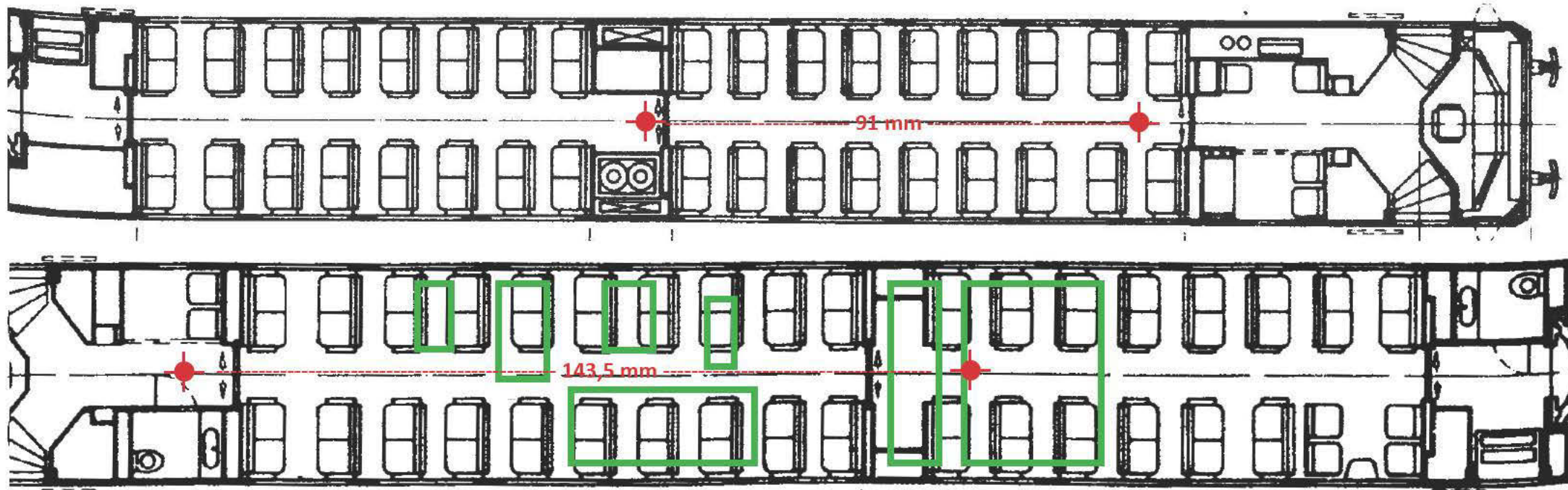
Plassering av seter for BM 92 (over) og styrevogn BS 92 og boring av hull til understell. Plassering av understellsdetaljer er merket med grønt. Skala 1:87
