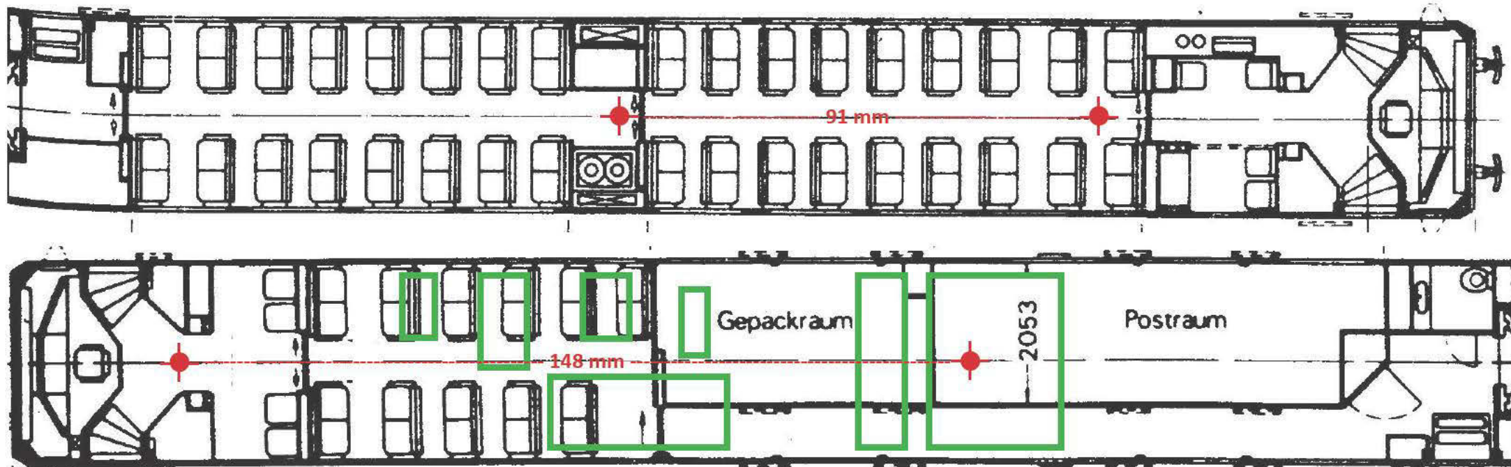
Plassering av seter for BM 92 (over) og styrevogn BDFS 92 og boring av hull til understell. Plassering av understellsdetaljer er merket med grønt. Skala 1:87
